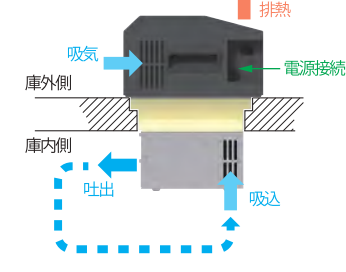
冷却ユニット模式図
