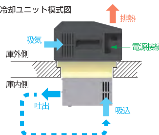
冷却ユニット模式図
