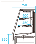
右側側面図
