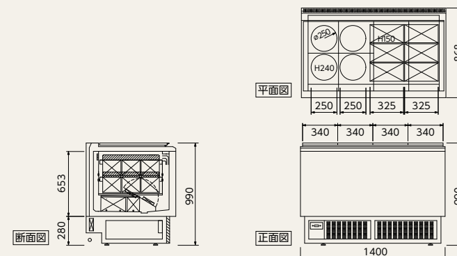
外径図
