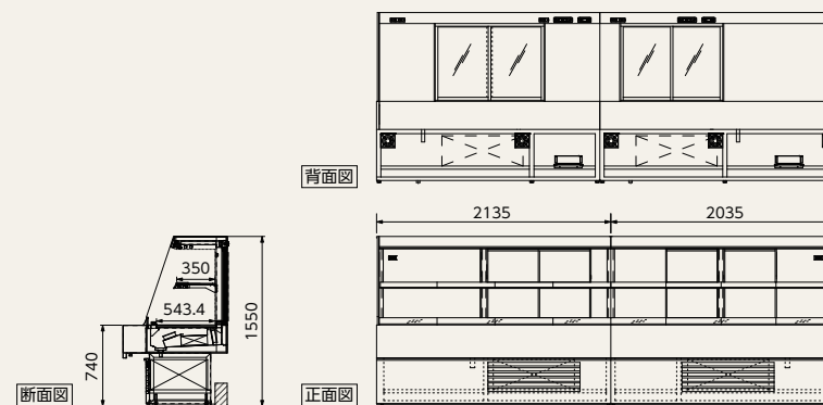
外径図
