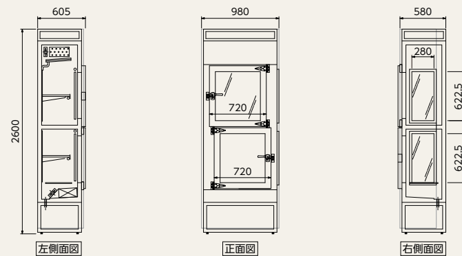
外径図
